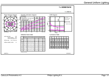
LEDBulb E27 ST64 400lm
